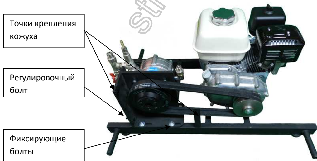
Рис.10 Регулировка ремня редуктора
