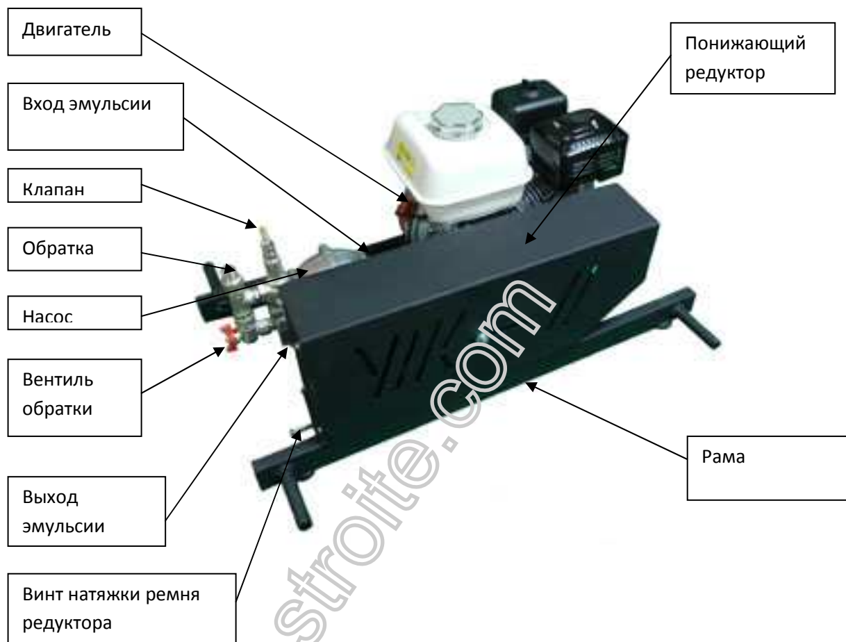
Рис. 3 Внешний вид гудронатора
