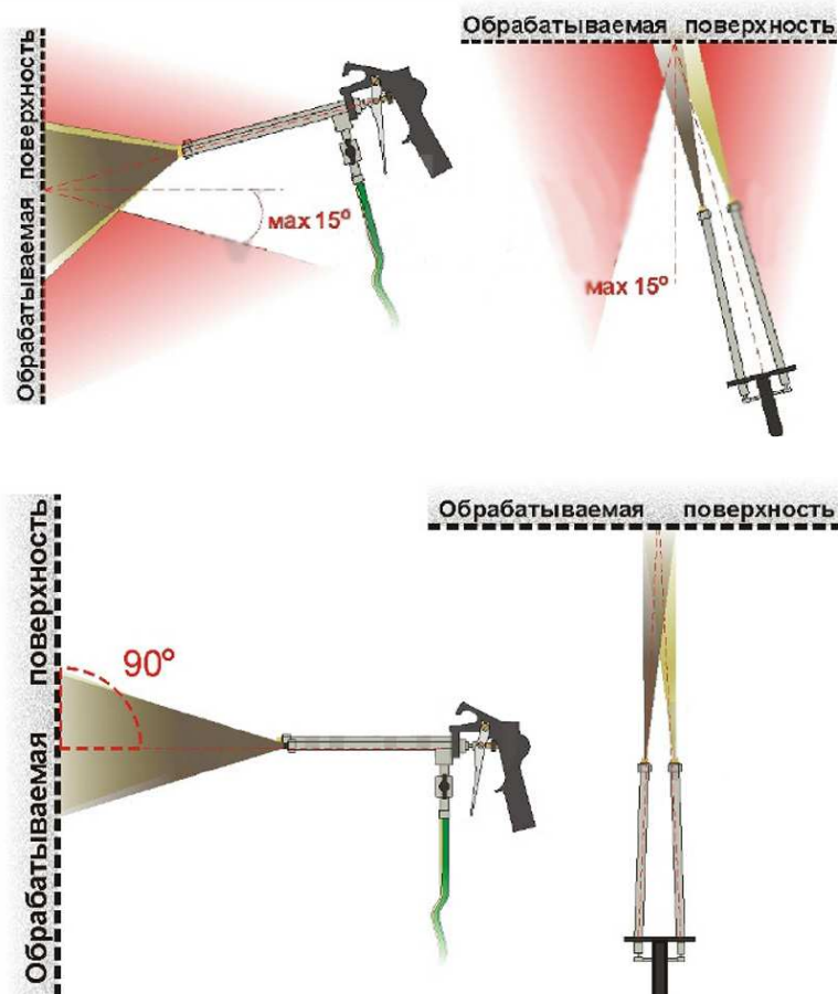
Рис.13 Нанесение жидкой резины
