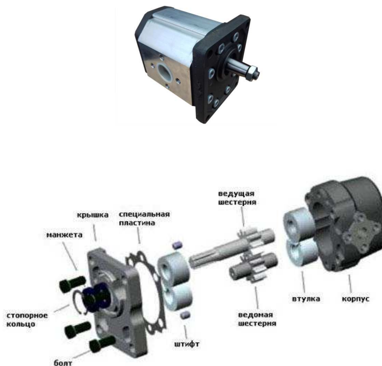
Рис. 4.1 Насос для подачи компонента «А»
