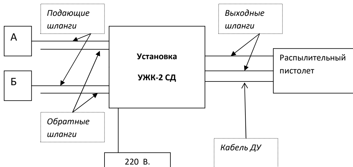
Рис.1 Схема подключения установки
