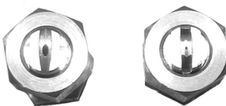
Рис.7 Рабочее положение форсунок.
