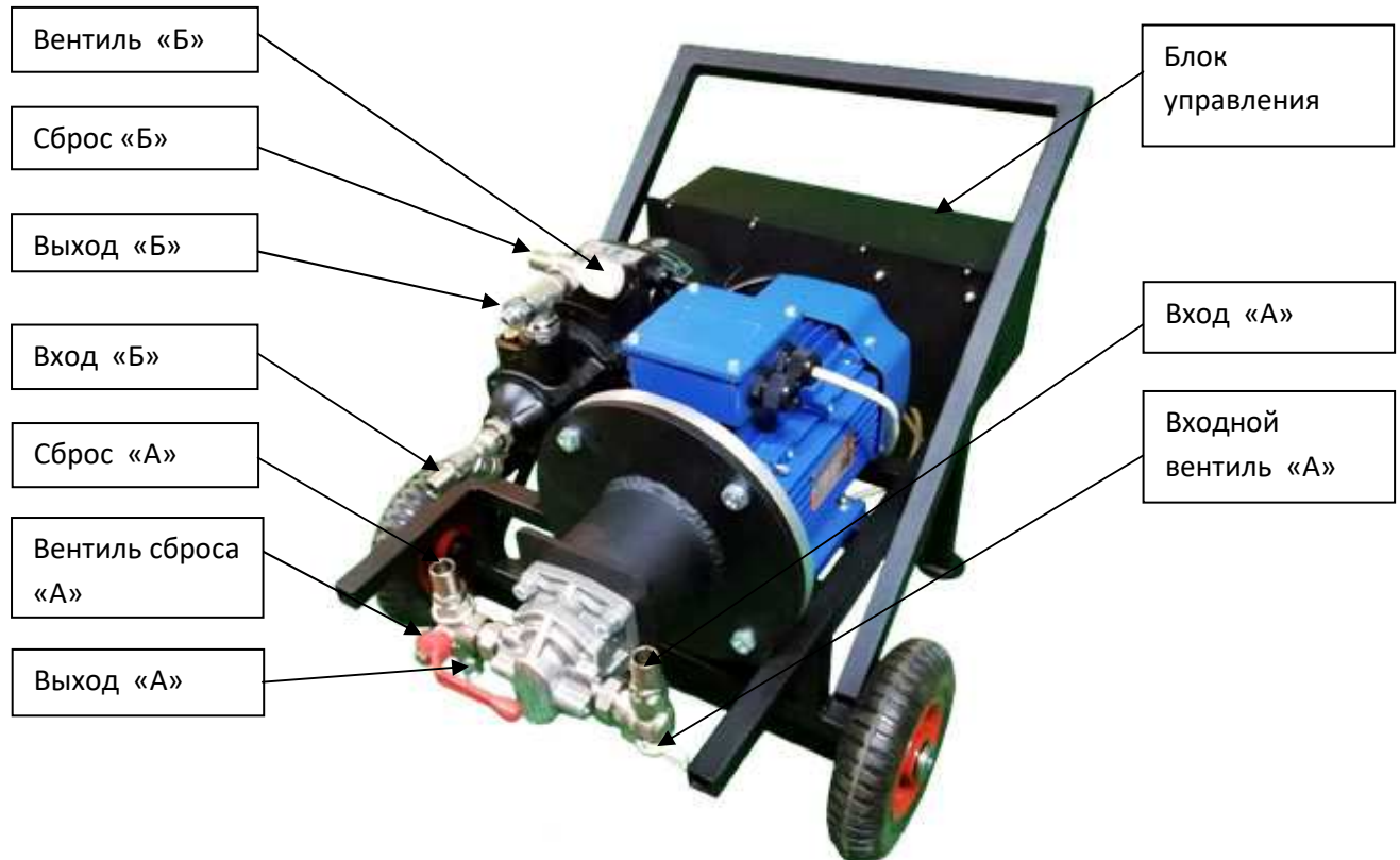
Рис.3 Внешний вид установки.
