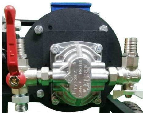
Рис.12.1. Открытое положение входного вентиля и вентиля сброса «А»
