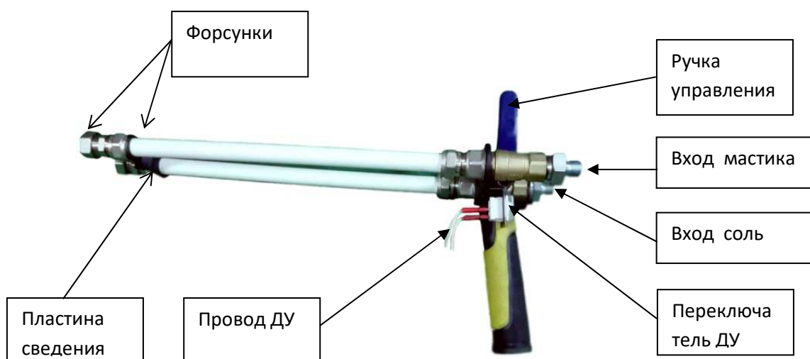
Рис.6 Основные элементы распылительного пистолета
