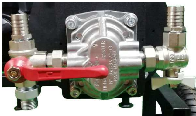
Рис.12.2. Закрытое положение вентиля сброса «А»
