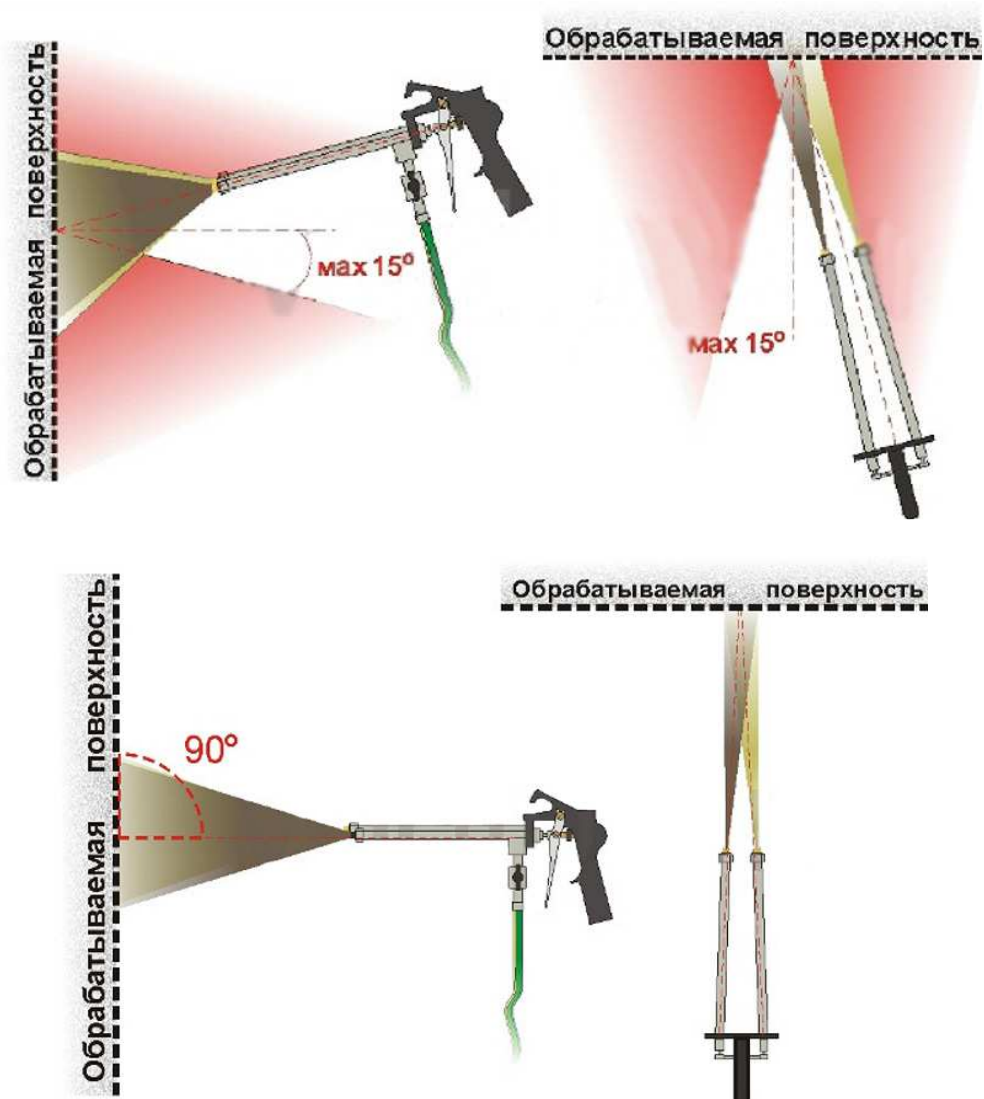
Рис.13 Нанесение жидкой резины
